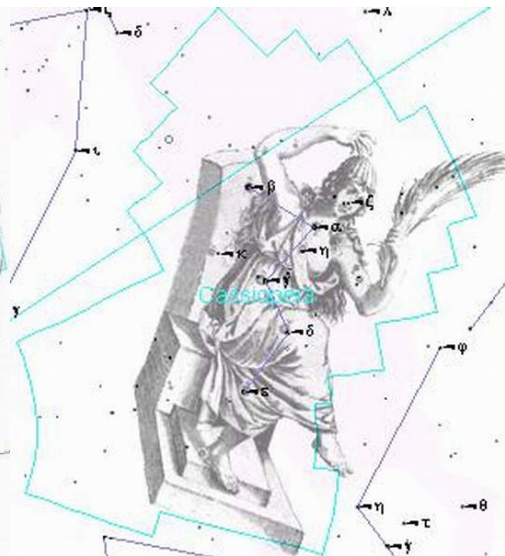
Созвездие Кассиопея
